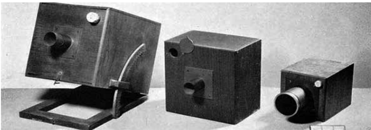
Камеры Генри Фокса Тальбота с отверстием для осмотра
