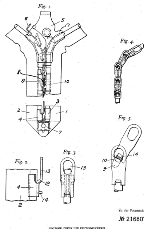
Чертёж из патента Гидеона Сундбэка 1909 года
