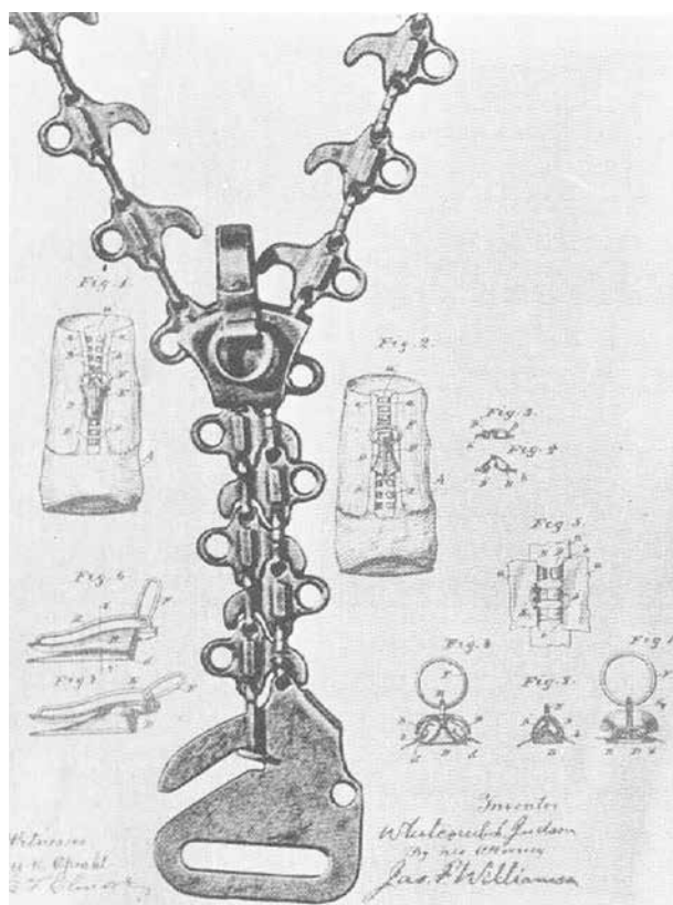
Чертёж первой версии застёжки-молнии Уиткомба Джадсона
